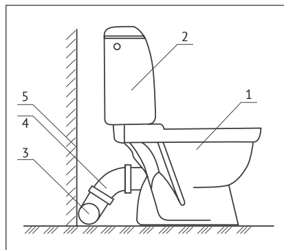
Схема установки унитаза с горизонтальным спуском
