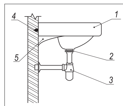
1 – Умывальник; 2 – Мебельная тумба; 3 – Сифон гофрированный; 4 – Канализационная труба; 5 – Крепежный болт
