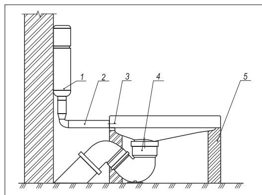
1 – бачок, 2 – подводящий патрубок, 3 – унитаз, 4 – колено, 5 – основание
