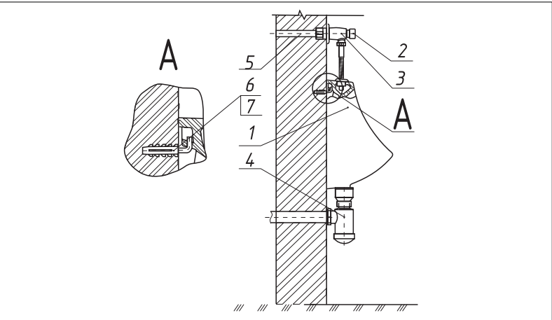
Схема монтажа писсуара ЛЮКС
