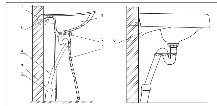
Схема установки умывальника на пьедестал/кронштейны
