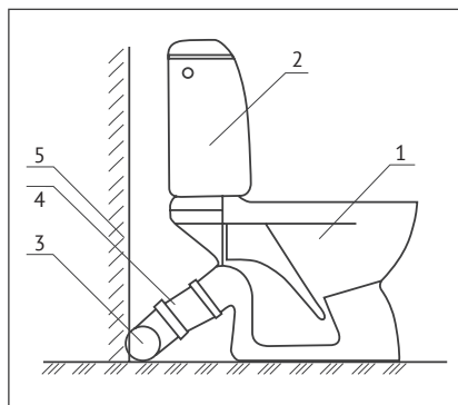
Схема установки унитаза с косым спуском
