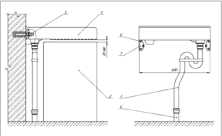
Схема установки умывальника над стиральной машиной
