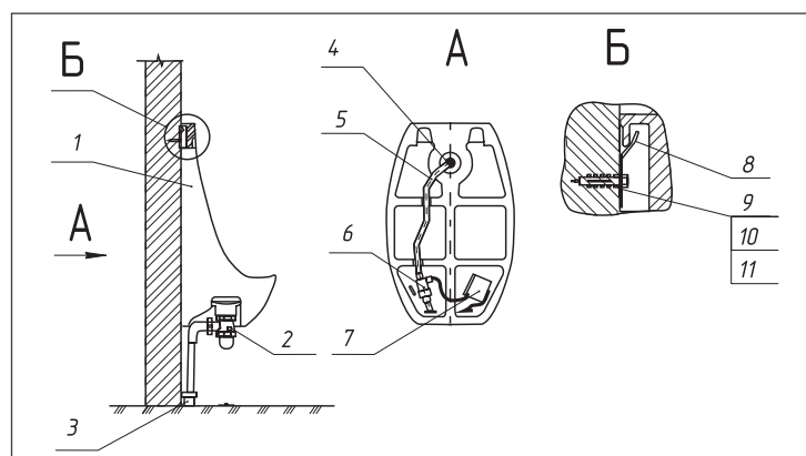
1 – Писсуар 2 – Сифон 3 – Ввод в канализацию 4 – Слив 5 – Гибкий шланг 1/2" 6 – Электромагнитный клапан 7 – Блок управления 8 – Кронштейн 9 – Саморез 10 – Шайба 11 – Дюбель
