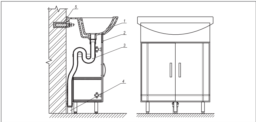
Схема установки умывальника на мебельную тумбу
