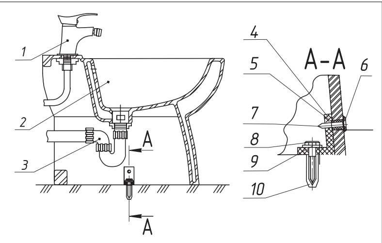
Схема монтажа биде
